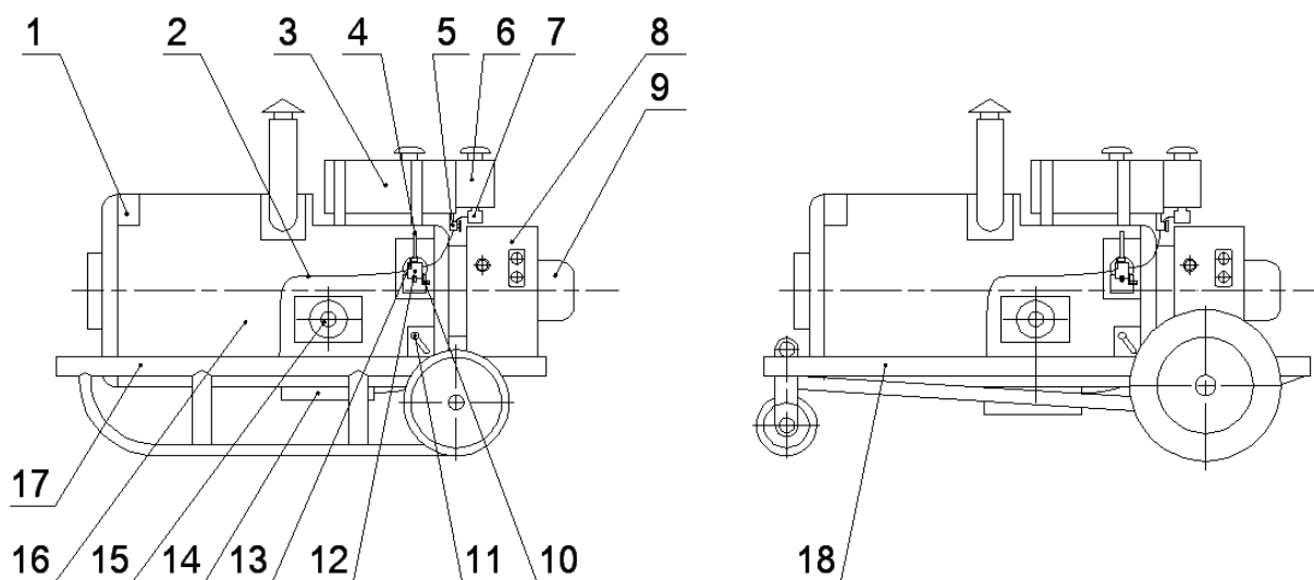
Рисунок 1 - Общий вид подогревателя.
